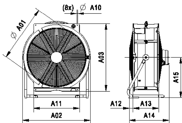
Figuur 2: Mobiele ventilator met 3- stappenregelaar
