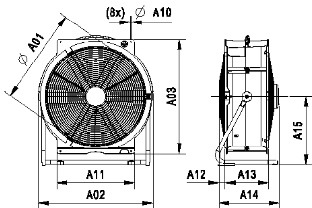
Figuur 1: Standaard mobiele ventilator
